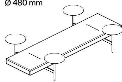
Nia wall L 3000/2370 P 600/1100 H 400/602 mm Ø 480 mm
